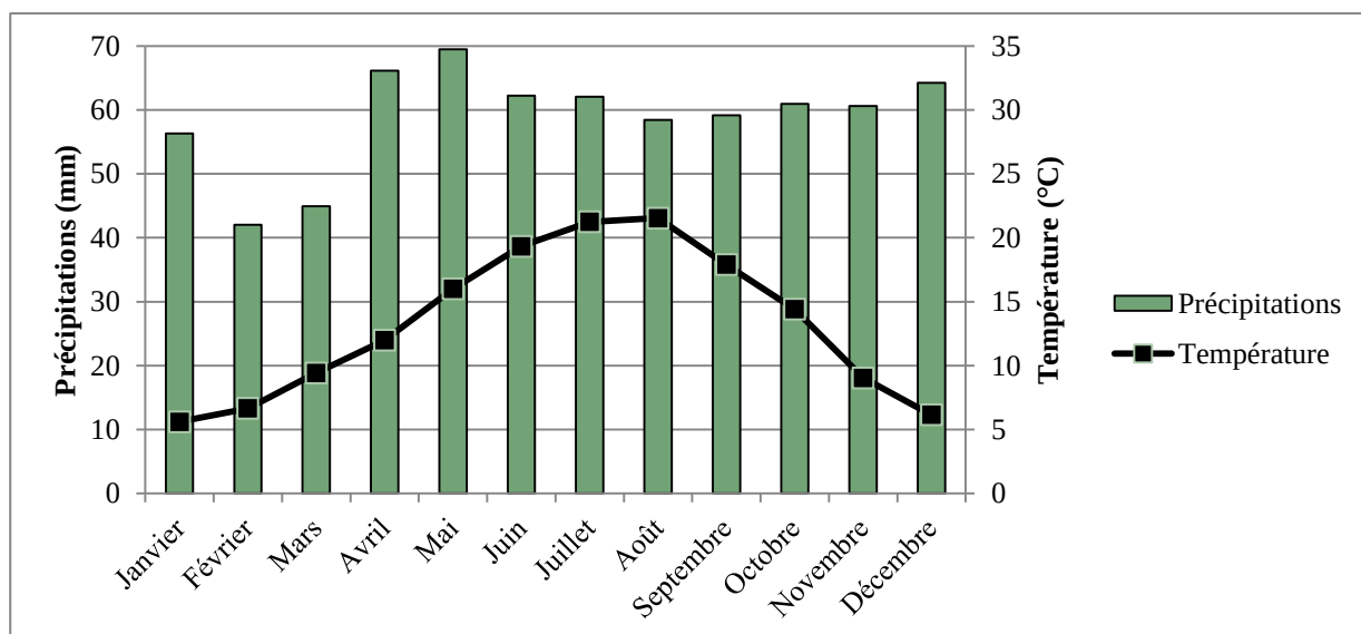
Figure 4: Diagramme ombrothermique sur la base de la formule de Gaussen : P=2T (données Météo France, station de Auch Lamothe, moyenne de 1992 à 2011)
