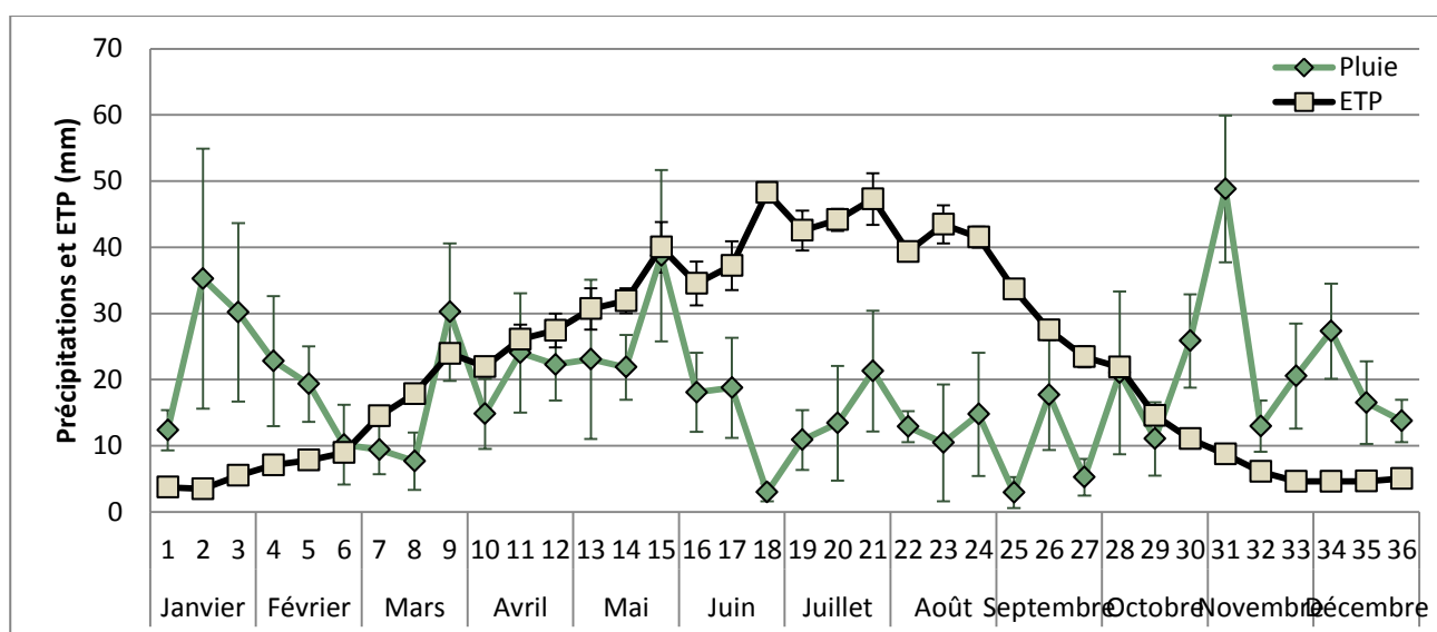
Figure 5: Précipitations et évapotranspiration potentielle (ETP) : moyenne interannuelle des cumuls par décade (données INRA de la station météo de la Hourre, de janvier 2009 à juillet 2013 inclus). Les barres verticales représentent l'erreur standard.
